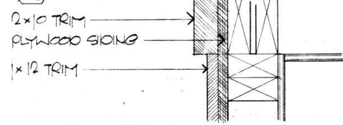
5 A-3 JAMB AT BLIND DOOR
