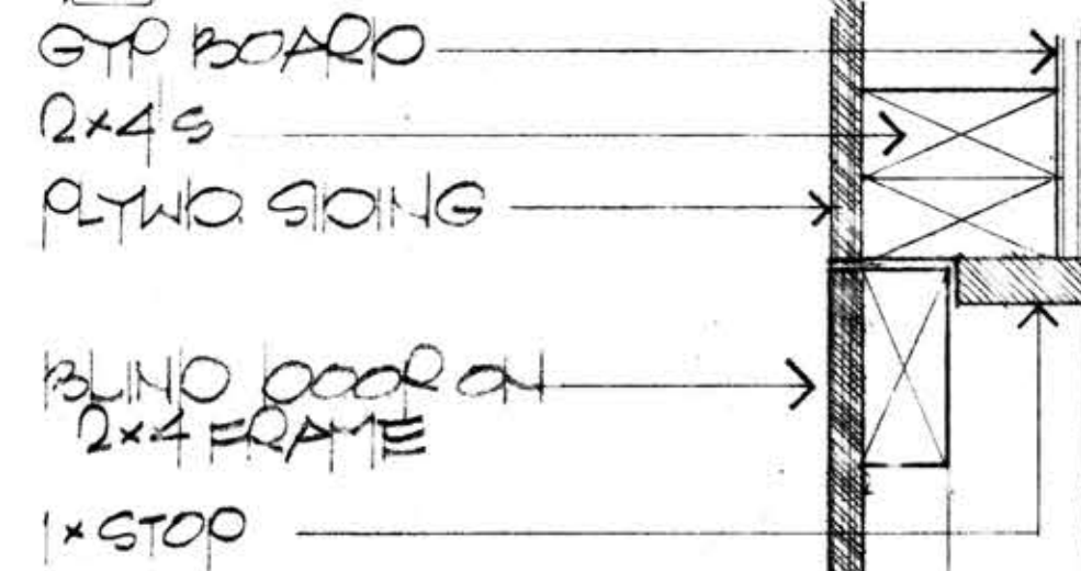
5 A-3 JAMB AT BLIND DOOR
