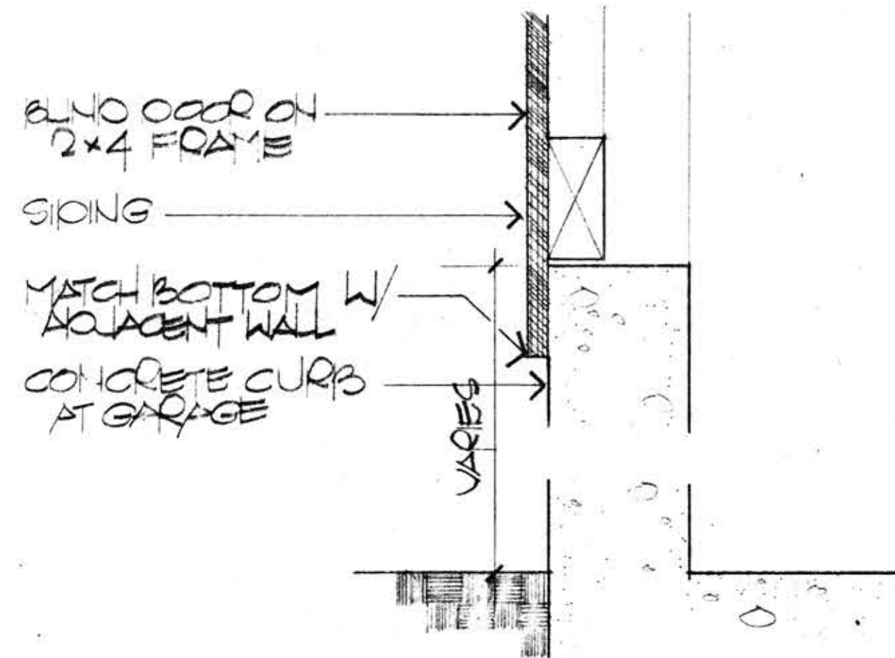
4 A-3 SILL AT BLIND DOOR
