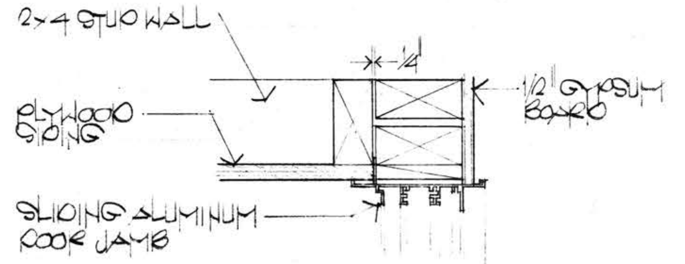
8 A-3 ALUMINUM DOOR JAMB
