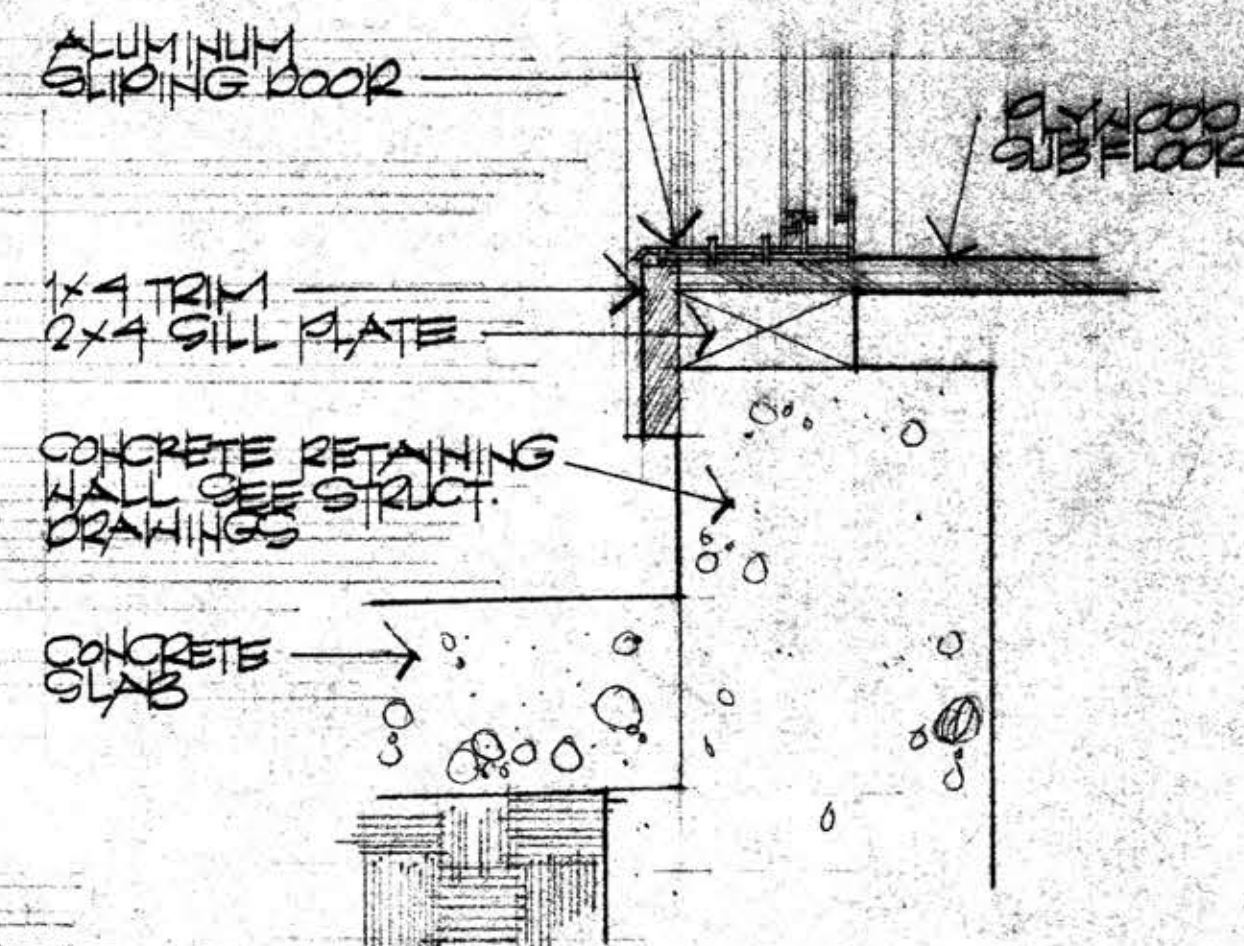
15 SILL-SLIDING DOOR
