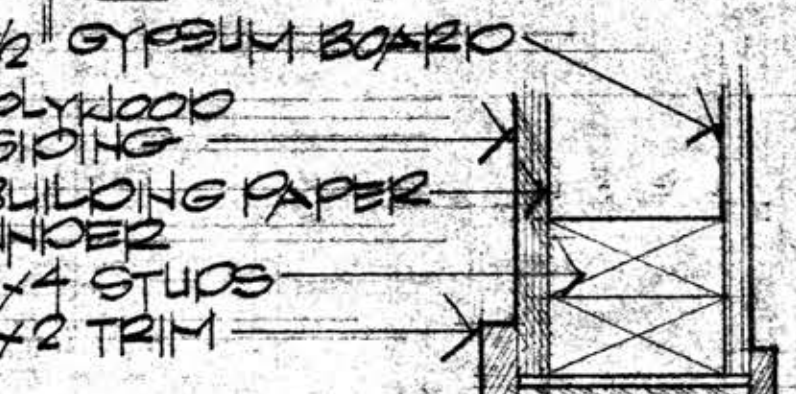
13 JAMB
