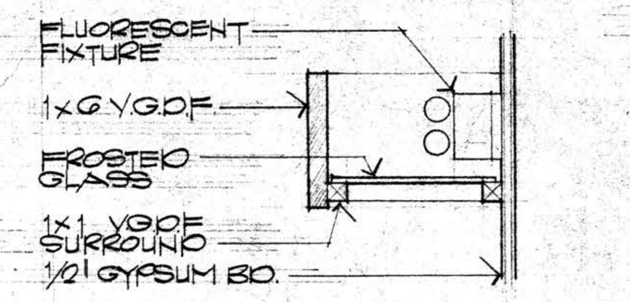
17 LIGHT VALANCE
