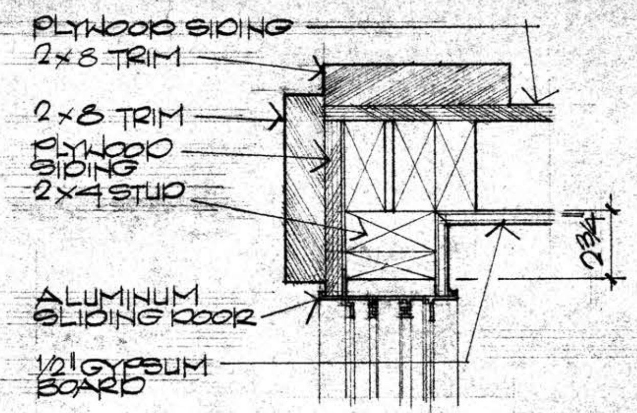
14 JAMB
